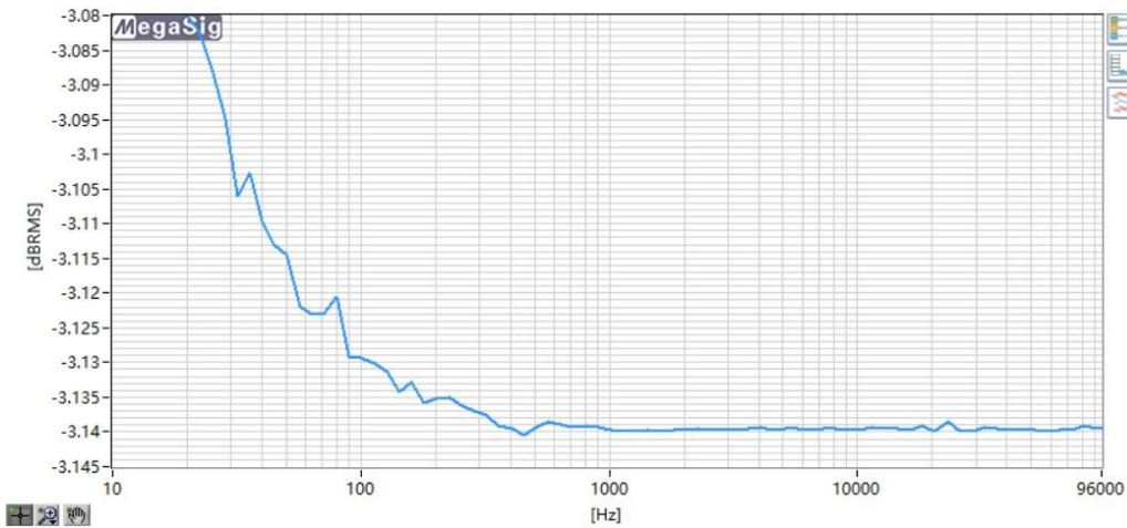
fs=192kS/s(20Hz-95kHz)
